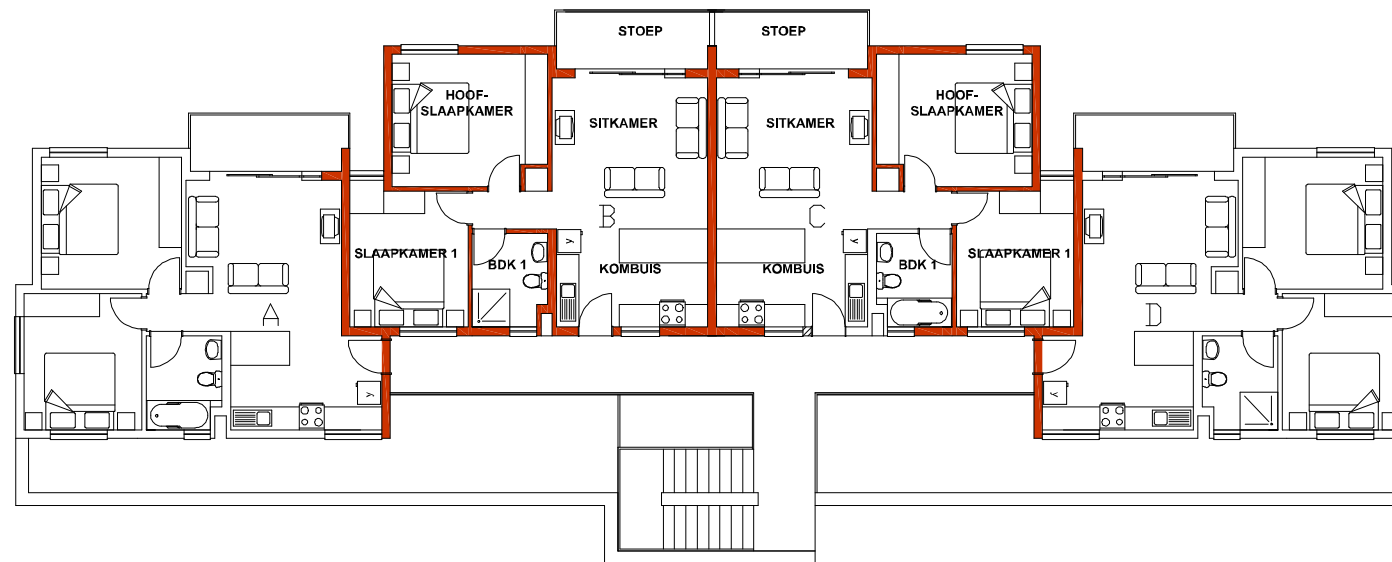
TWEESLAAPKAMER WOONSTEL BLOK SKAAL 1:200
